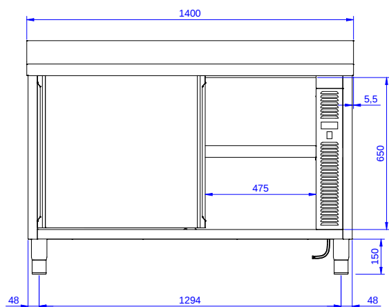
Alzado
